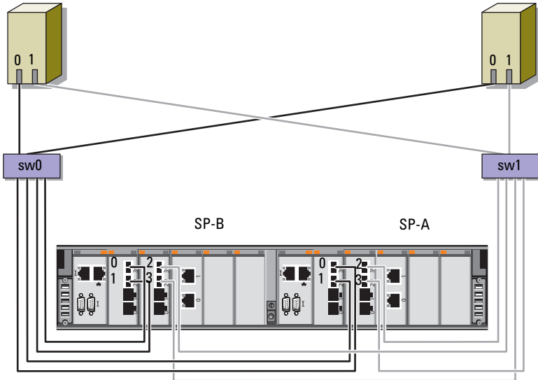
图 3-3. 在 SAN 连接的光纤信道群集中布线
